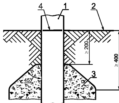
1 — опора; 2 — поверхность покрытия игровой площадки; 3 — фундамент; 4 — базовая отметка заглибления
