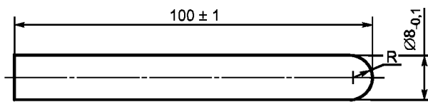
Рисунок Г.12 — Стержень-палец А (малый)
