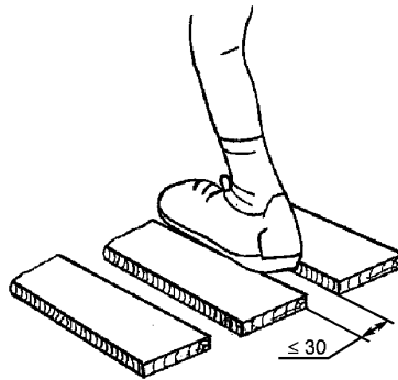
Рисунок 8 — Ширина зазоров на поверхностях с наклоном до 45°
