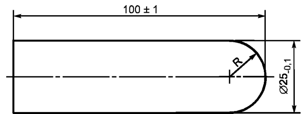
Рисунок Г.13 — Стержень-палец Б (большой)
