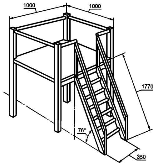
Рисунок А.1 — Платформа с лестницей
