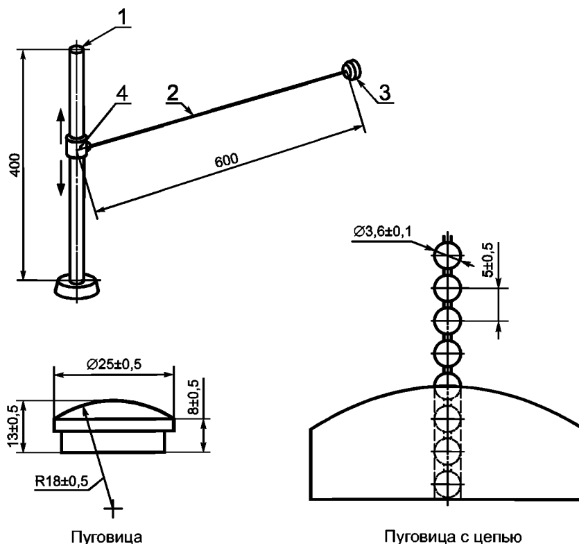
1 — стойка; 2 — цепь; 3 — пуговица из полимерного материала; 4 — втулка; R — радиус лицевой поверхности пуговицы
